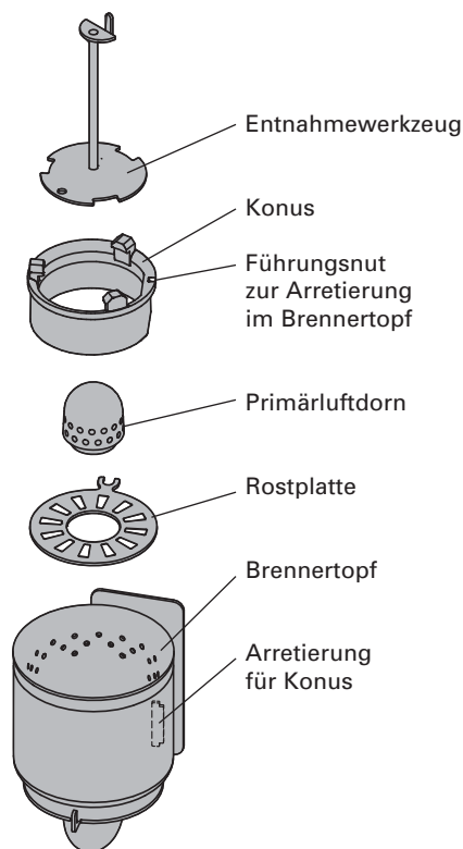
Abb. 128 Brennertopf
